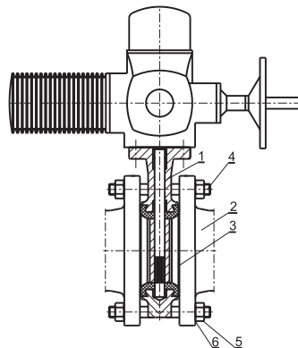
Схема монтажа
